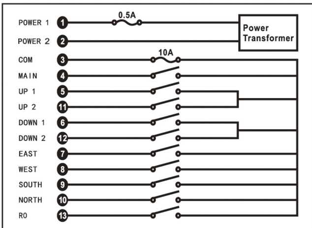
Q602 Wiring Diagram
