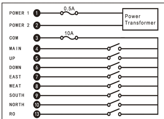
Q600 Wiring Diagram
