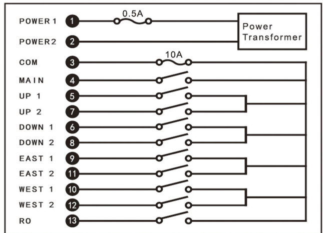
Q404 Wiring Diagram
